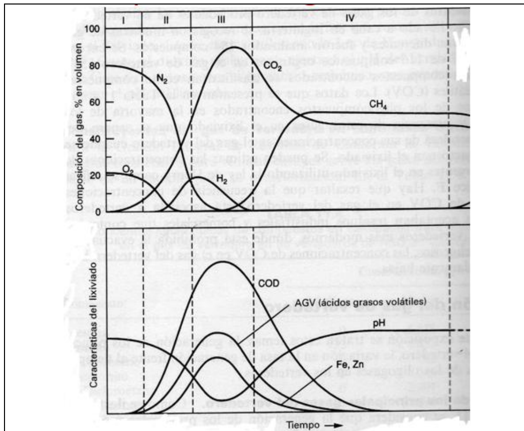
Figura 7. Comportamiento de gases y lixiviado en un relleno sanitario
